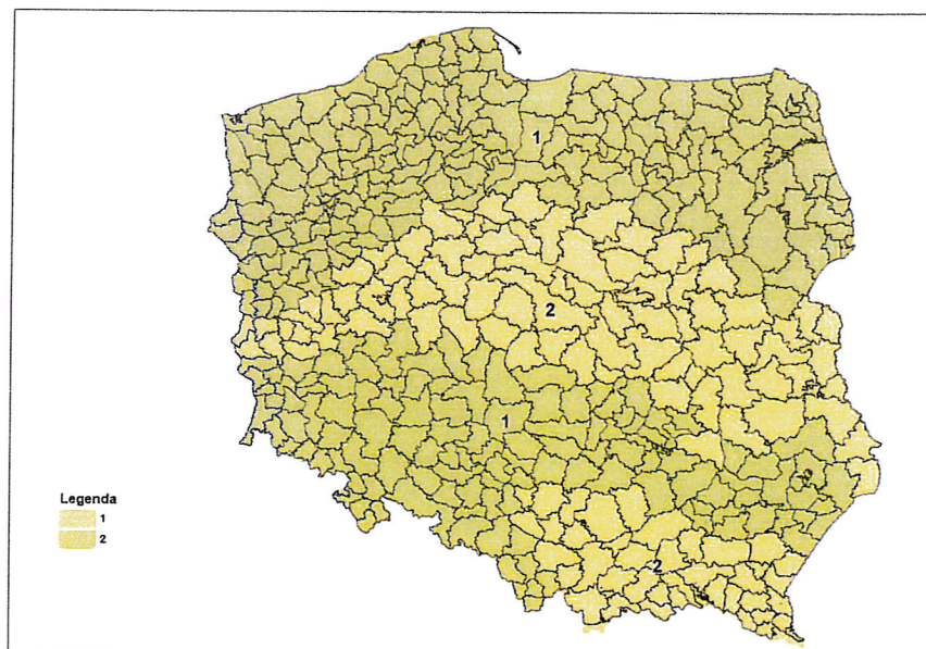
Rys. 2. Potencjalny zasięg występowania Świerka pospolitego
