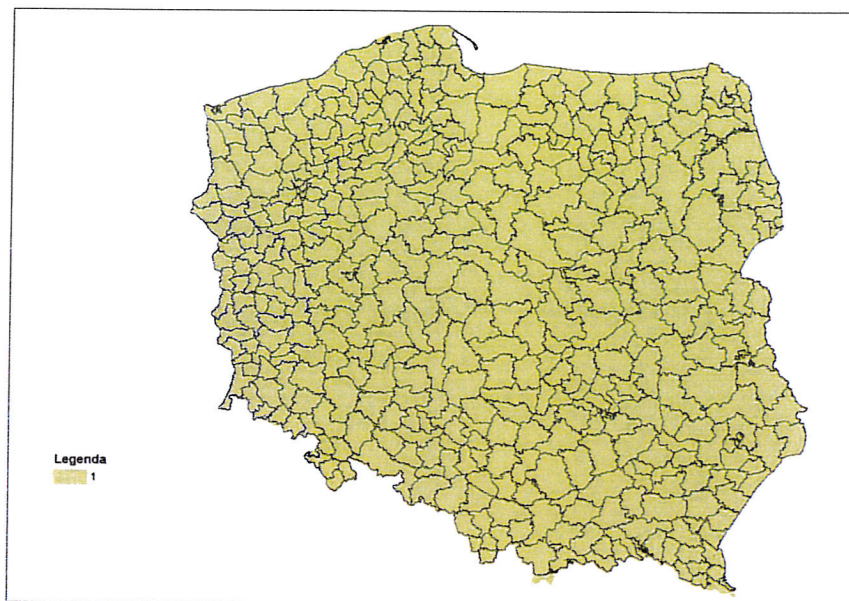
Rys. 1. Potencjalny zasięg występowania Sosny zwyczajnej
