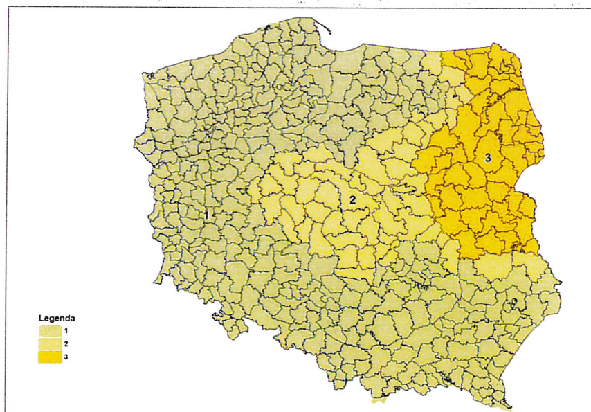
Rys. 4. Potencjalny zasięg występowania Buki zwyczajnego
