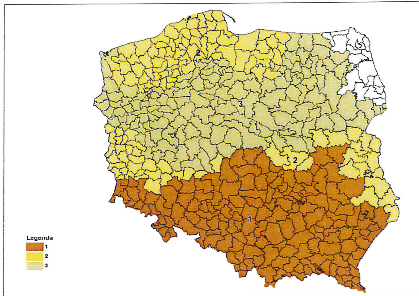
Rys. 5. Potencjalny zasięg występowania Jodły pospolitej
