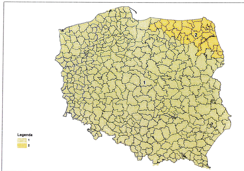
Rys. 3. Potencjalny zasięg występowania Dębu bezszypułkowego
