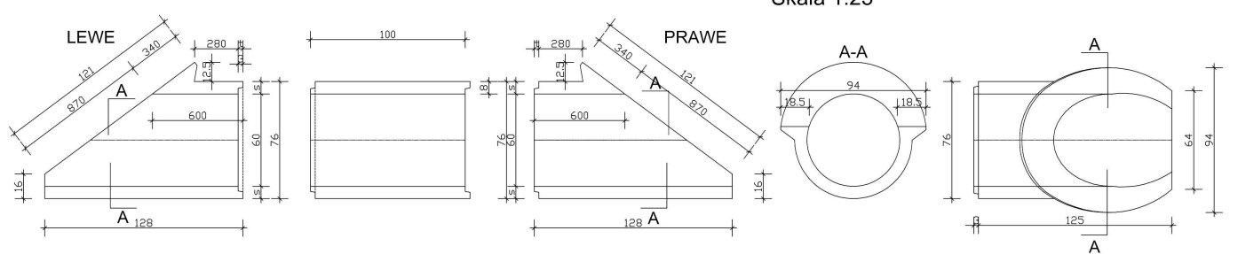
KOŁNIERZOWE ZAKOŃCZENIE PRZEPUSTU Dw=600 Skala 1:25
