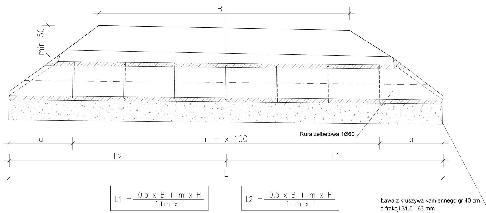
KOŁNIERZOWE ZAKOŃCZENIE PRZEPUSTU Dw=600 Skala 1:25
